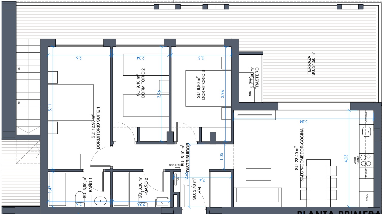
PLANTA PRIMERA
