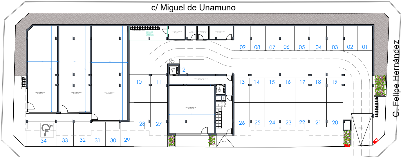
PLANTA 0
